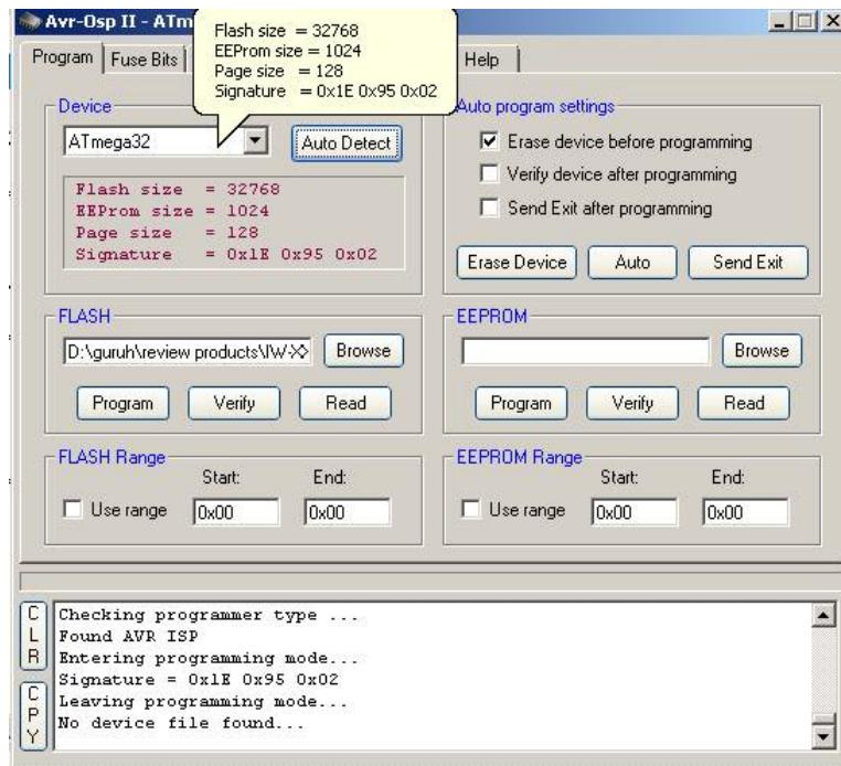
Gambar 12. Auto detectAvrOspII.
